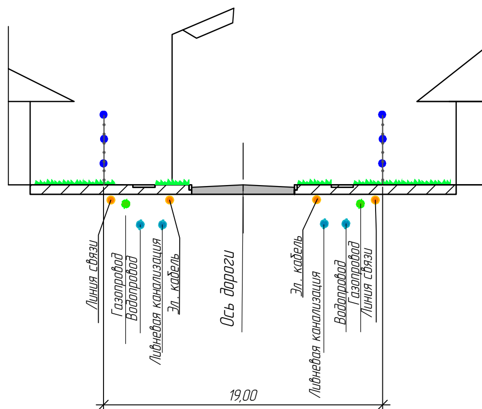
Разрез 1-1.
